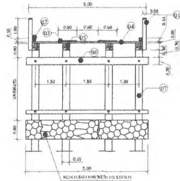
SEÇÃO TRANSVERSAL - PILARES DE CABEÇEIRA ESCALA - 1:24
