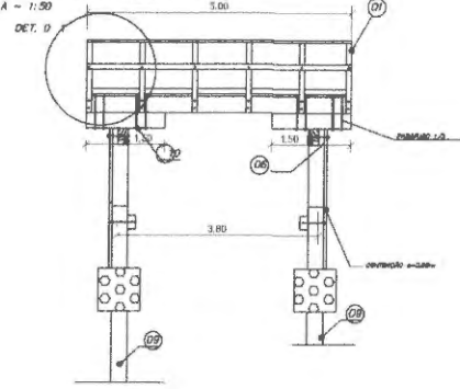
SEÇÃO LONGITUDINAL - PONTE ESCALA - 1:50
