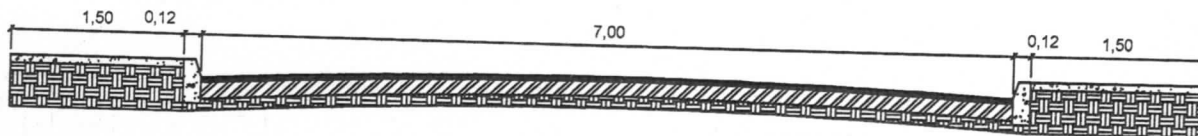
PERFIL TRANSVERSAL
