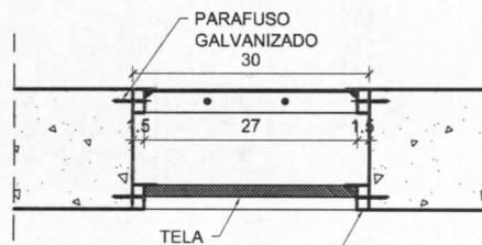
SEÇÃO 1-1 ESC. 1/10
