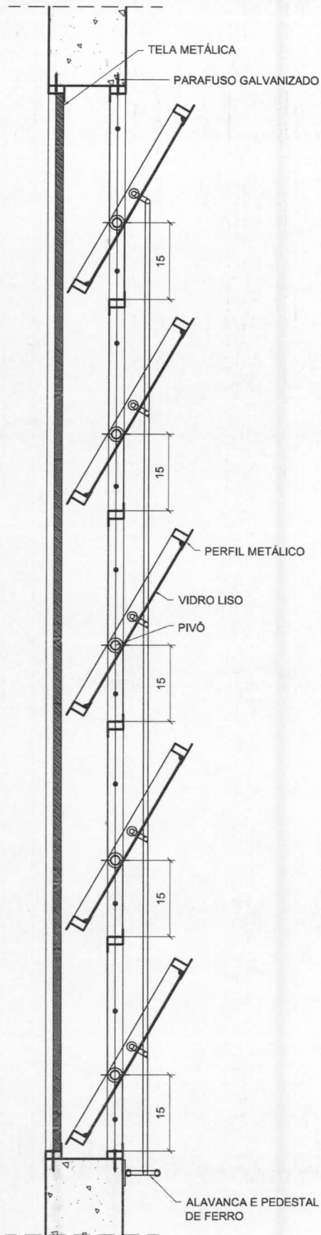
SEÇÃO 1-1 ESC. 1/10
