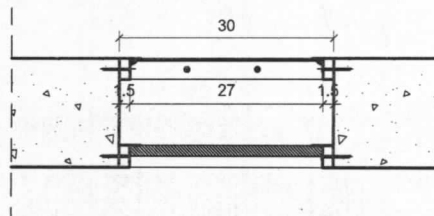
SEÇÃO 1-1 ESC. 1/10
