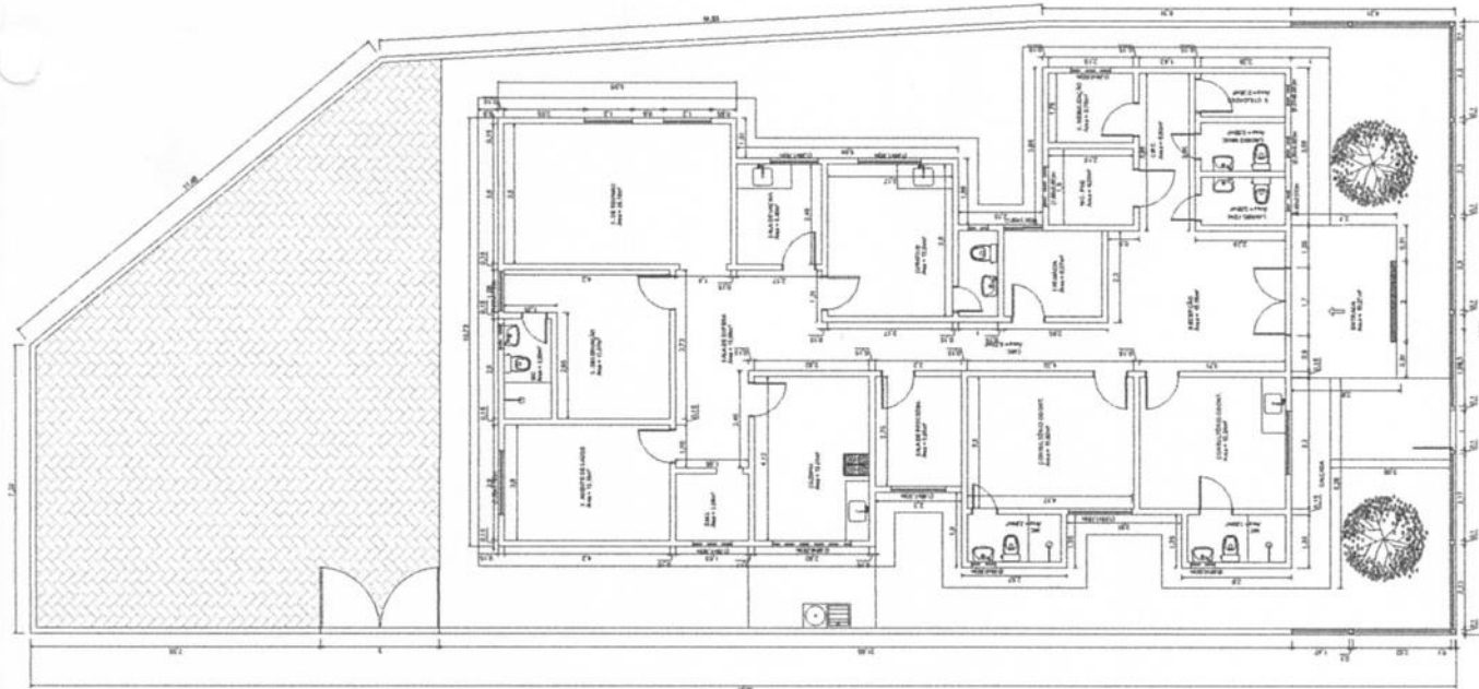
PLANTA DE COBERTURA ESCALA 1:50
