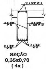
DET. FERRAGEM DO PAINELÃO
