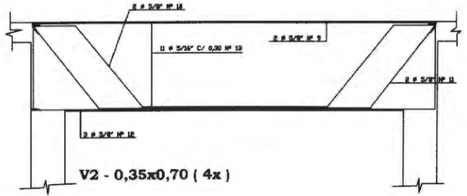
SEÇÃO 0,35x0,70 (4x)
