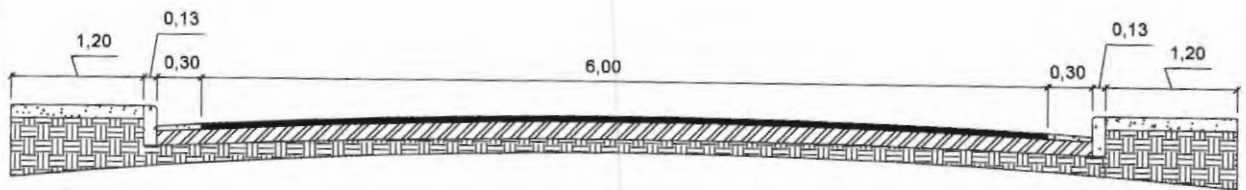
PERFIL TRANSVERSAL
