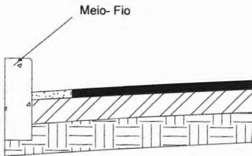
Detalhe "A"
